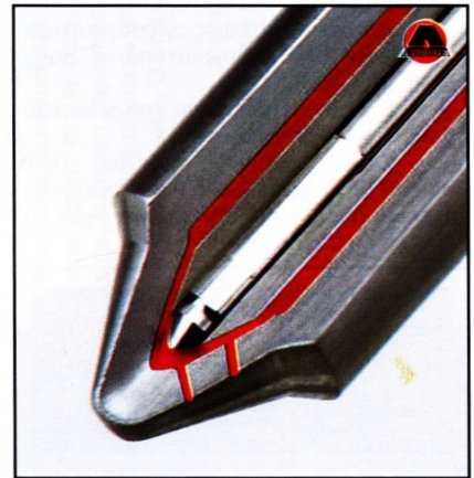
1. Впускная камера. 2. Корпус форсунки. 3. Гайка распылителя. 4. Проставка. 5. Распылитель. 6. Игла распылителя. 7. Полость распылителя. 8. Накидная гайка для соединения с трубопроводом высокого давления. 9. Фильтр. 10. Штуцер дренажной системы. 11. Прокладка регулирования давления впрыска. 12. Канал высокого давления. 13. Пружина. 14. Нажимной штифт.
