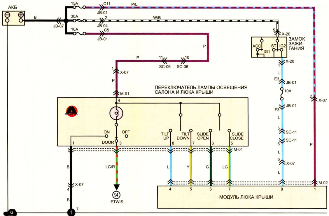
M-01 ПЕРЕКЛЮЧАТЕЛЬ ЛАМПЫ ОСВЕЩЕНИЯ САЛОНА И ЛЮКА КРЫШИ
