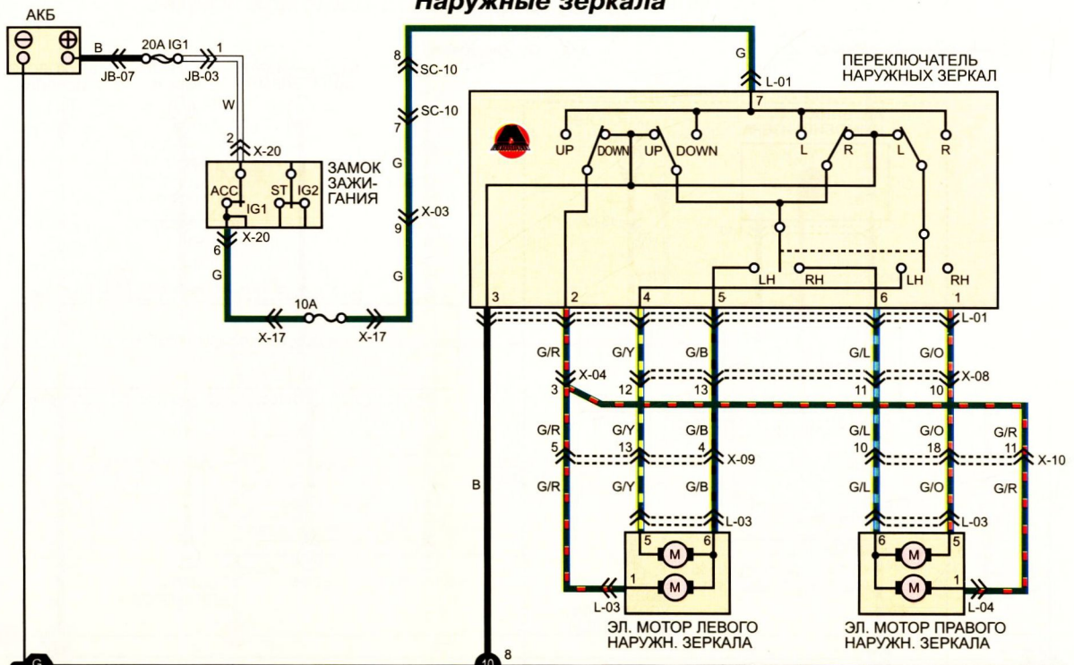
L-01 ПЕРЕКЛЮЧАТЕЛЬ НАРУЖНЫХ ЗЕРКАЛ
