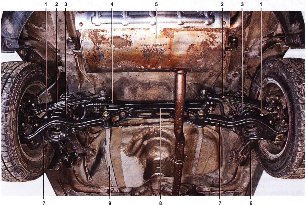
Вид снизу автомобиля 2WD (задняя часть): 1 — амортизатор задней подвески; 2 — верхний поперечный рычаг задней подвески; 3 — пружина задней подвески; 4 — стабилизатор поперечной устойчивости; 5 — глушитель; 6 — продольный рычаг задней подвески; 7 — нижний поперечные рычаги задней подвески; 8 — задний подрамник; 9 — топливный бак
