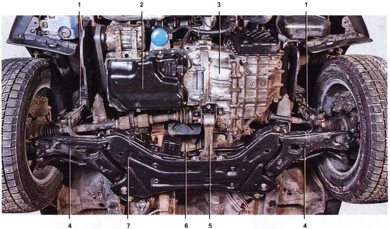
Вид снизу автомобиля 2WD (передняя часть со снятым брызговиком двигателя): 1 — стойка передней подвески; 2 — двигатель; 3 — коробка передач (АКП); 4 — рычаг передней подвески; 5 — задняя опора силового агрегата; 6 — рулевой механизм; 7 — передний подрамник
