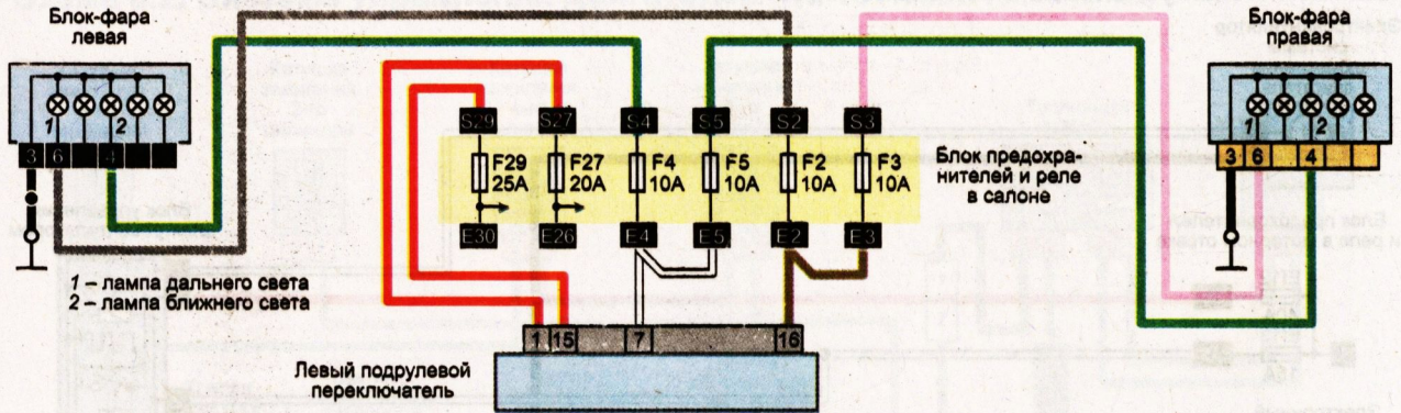
Схема 10. Габаритное освещение, фонарь освещения номерного знака
