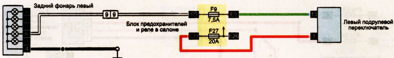
Схема 12. Задний противотуманный фонарь
