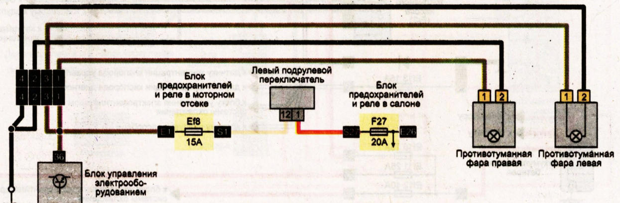
Схема 11. Противотуманные фары
