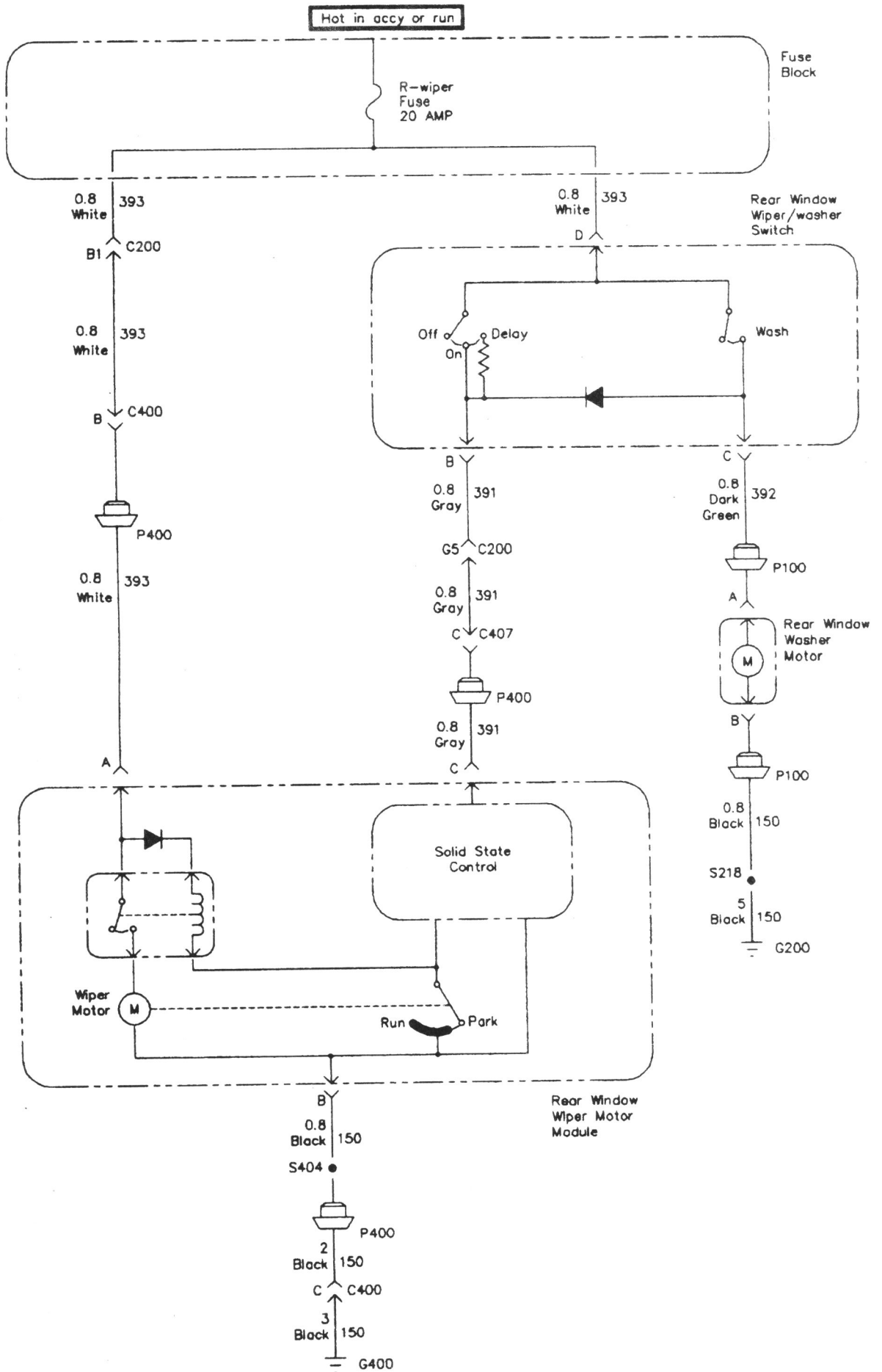
18 – Типичная схема электрической цепи стеклоочистителя/омывателя заднего стекла.
