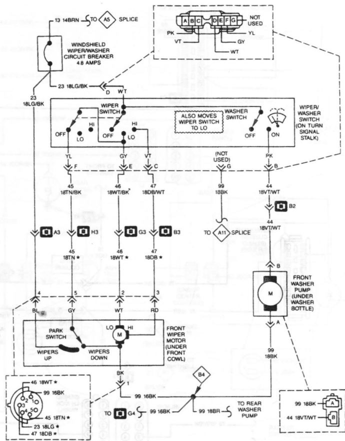
Электрическая схема стеклоочистителя ветрового стекла (непрерывного).
