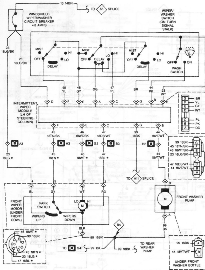
Электрическая схема стеклоочистителя ветрового стекла (прерывистого).
