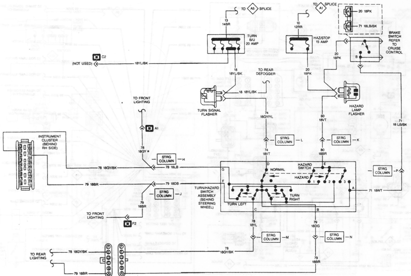
Электрическая схема стоп-сигналов, сигналов поворотов и аварийной сигнализации (модели типа "Commanche").
