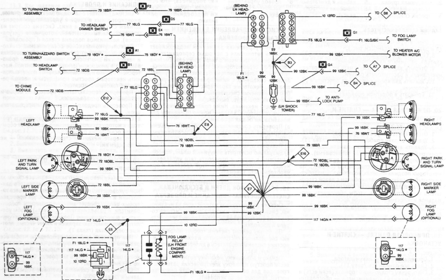
Электрическая схема передних огней (модели с четырьмя фарами).
