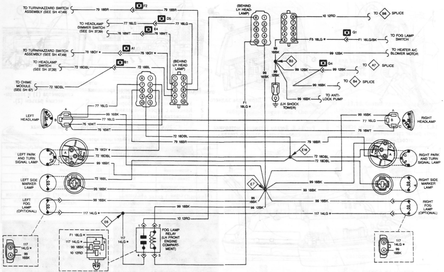
Электрическая схема передних огней (модели с двумя фарами).
