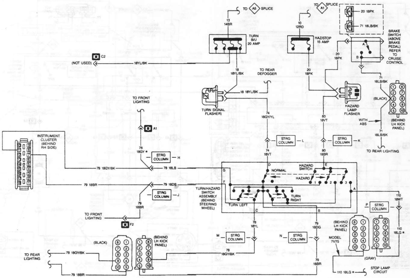
Электрическая схема стоп-сигналов, сигналов поворотов и аварийного сигнала (модели типа "Cherokee").
